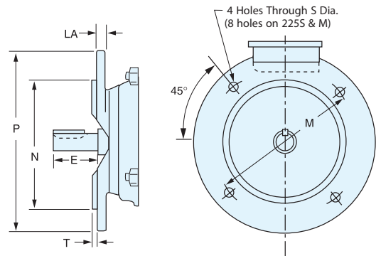
B5 FLANGE
