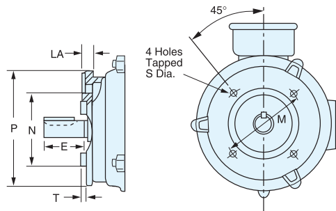
B14 FLANGE
